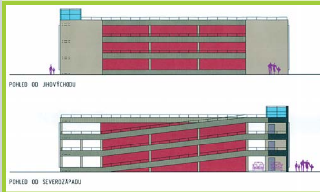
Pohledy ze dvou stran.
