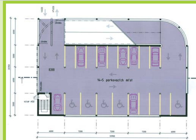
Přízemí s rozšířeným místem pro imobilní spoluobčany s bezbariérovým přístupem.
