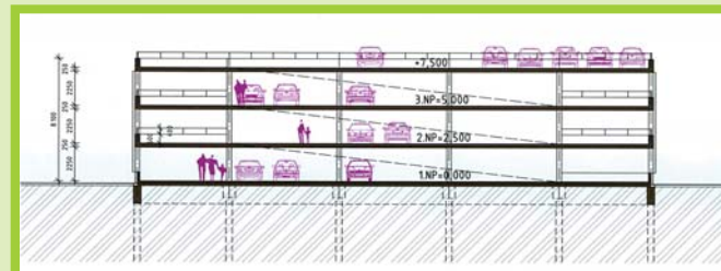
Technický průřez parkovištěm. Přízemí, dvě poschodí a parkoviště na střeše.
