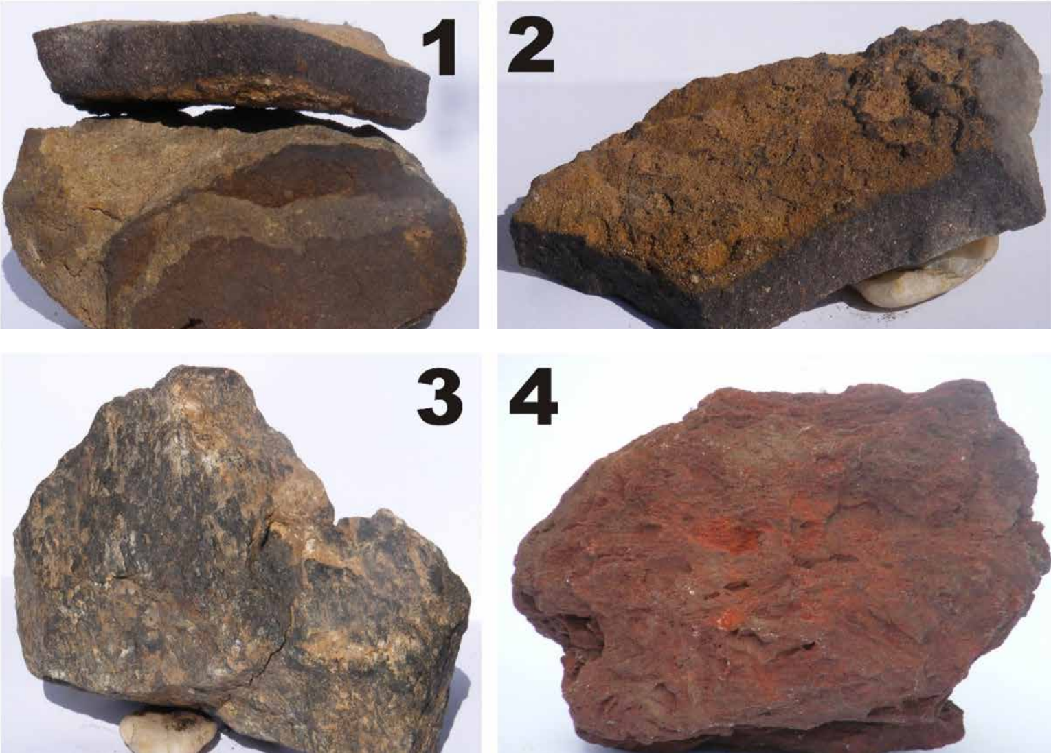
Obr. 2 Horniny z hlavního hřebene a jeho okolí s nadprůměrným obsahem železa 1, 2 – návrší Brda 3 – severní svah vrcholu Oberský 4 – sedlo pod vrcholem Rudovka
